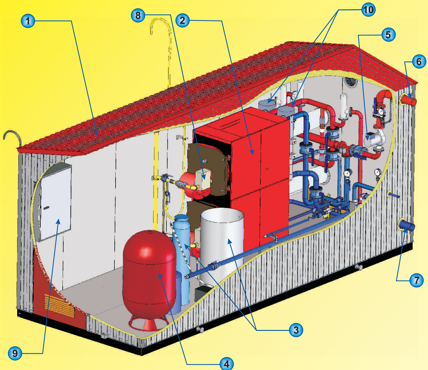
Установка котельная модульная УКТМ-400
