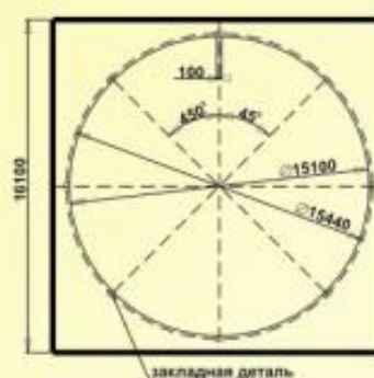
План фундамента
